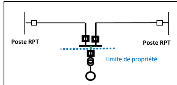
SCHÉMA 3 : Raccordement en coupure sur une liaison du RPT au niveau de l'Installation
